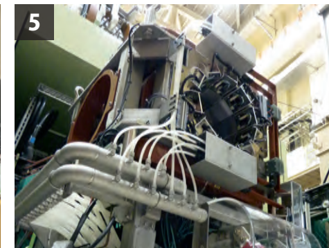
ミュオン実験装置 ミュオンビームラインの最下流に位置する装置。ビームライン に沿って導かれ、試料内部に撃ち込まれたミュオンが崩壊 する際に放出する陽電子をキャッチします。
