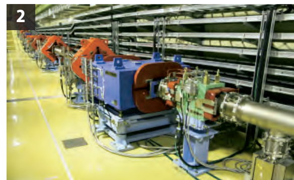
3GeV 陽子ビーム輸送ライン 超高真空のビームダクト内の 3GeV 陽子ビームを、地下に建設されたトンネル内を通して、300mほど離れた物質・生命科学実験施設まで導きます。
