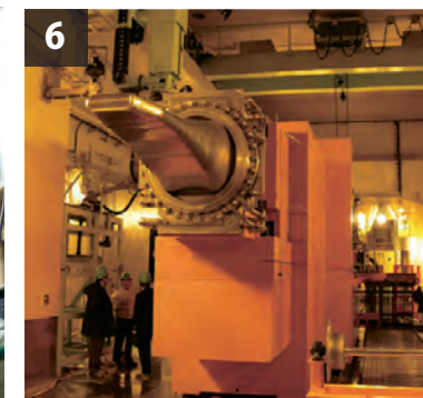
中性子生成用水銀ターゲット 中性子を発生させるための標的。水銀を内包 しており、水銀自体が循環し放熱する仕組み です。
